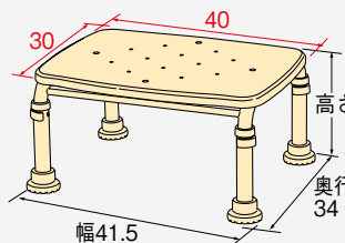
商品寸法図
