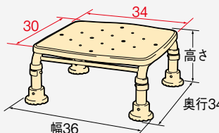
商品寸法図
