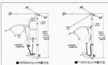
■F2RSKKセット外観寸法
